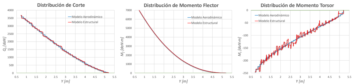
Figura 4: Redistribución de Cargas sobre el ala de una aeronave – Esfuerzos Integrados
